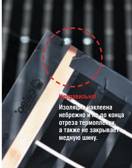
Рис. 14. Пример неправильной установки ПВХ изоляции
