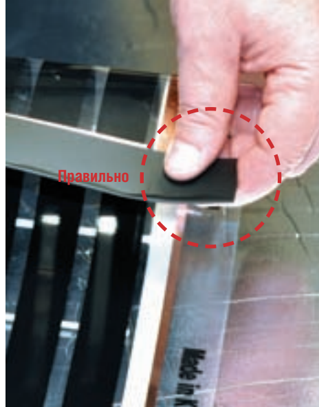
Рис. 12. Пример правильной установки ПВХ изоляции вдоль всей линии разреза термопленки
