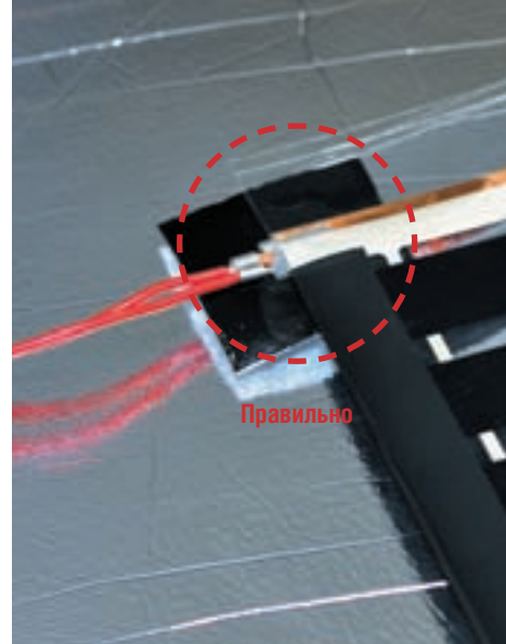
Рис. 18. Пример правильной установки нижнего листа битумной изоляции контактных зажимов
