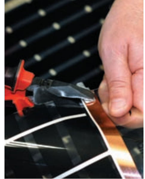
Рис. 10. Крепление контактного зажима к термоленке (обжатие плоскогубцами)
