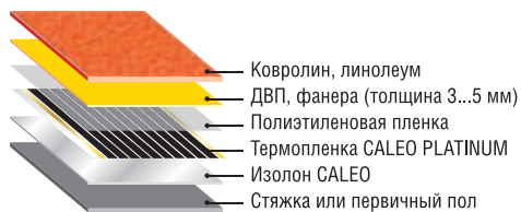
Рис. 4. Схемы монтажа теплого пола CALEO PLATINUM под ламинат, ковровлин, линолеум
