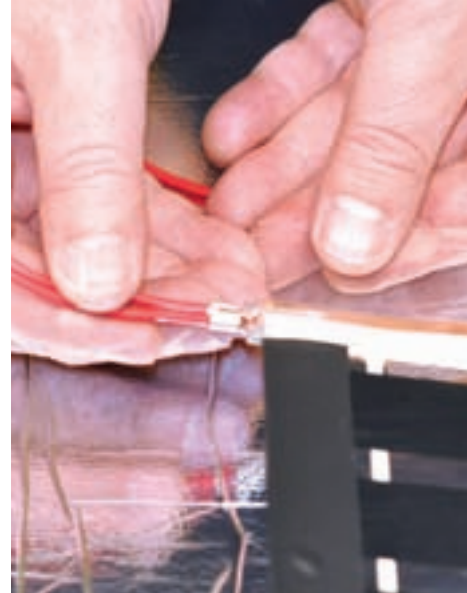
Рис. 15. Соединение монтажных проводов с контактным зажимом
