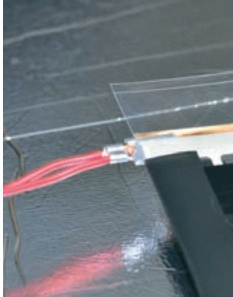
Рис. 17. Вид правильного подключения проводов к термопленке
